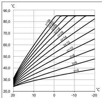
Coefficient de la courbe de chauffe
