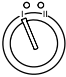
Reglerknopf in Stellung I ( P_{max} = 2/3 P_n )
